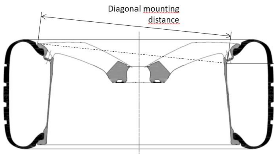
عجلة عادية
